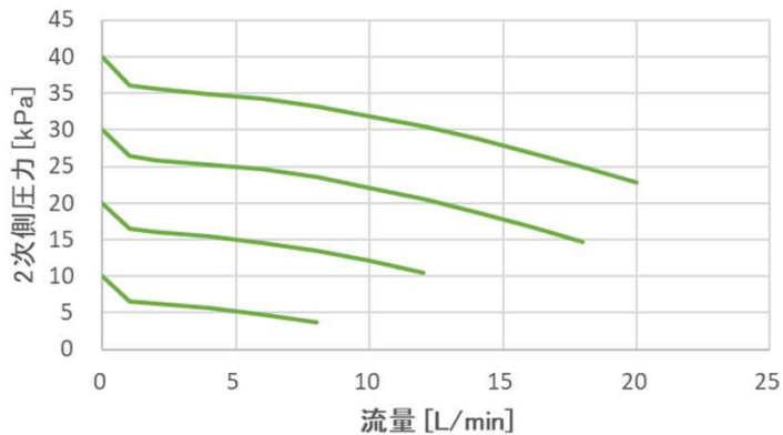
流量特性 (1次側圧力150kPa)
