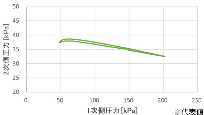
圧力特性 (流量5L/min)
