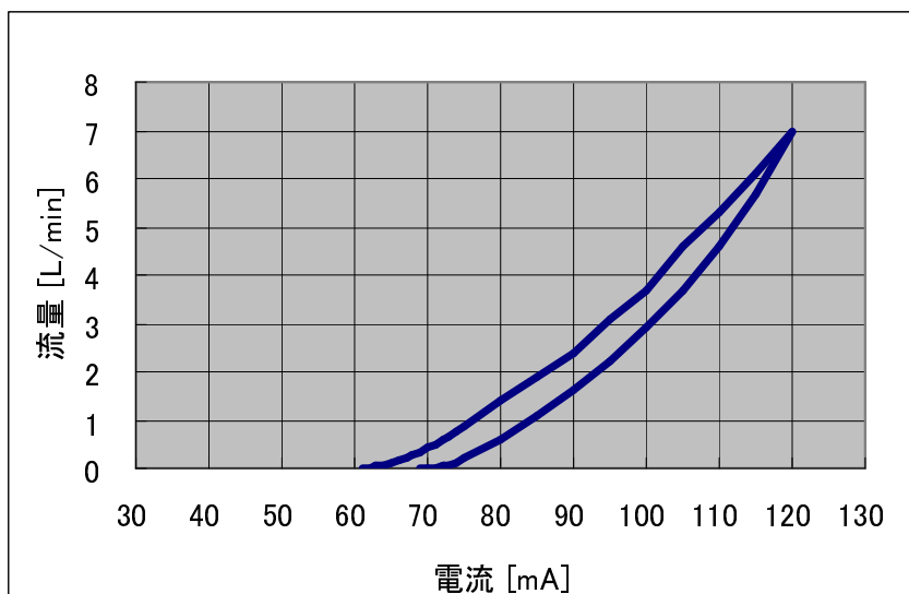
電流－流量特性例（室温）
