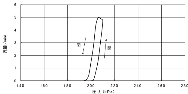
■泄压特性 ( VR1-B-M2-200 )
