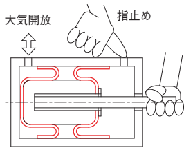
Fig.4 複動形引出の場合
