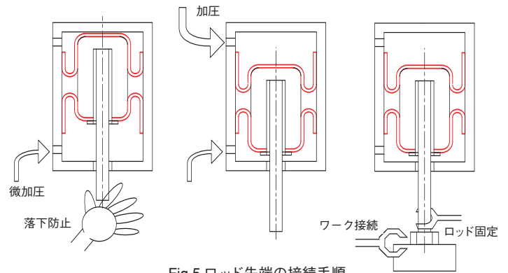
Fig.5 ロッド先端の接続手順
